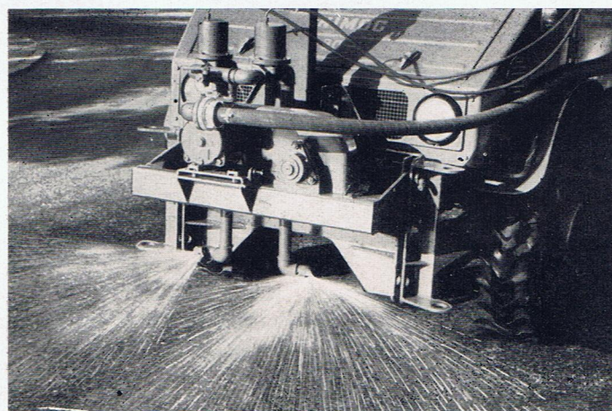
WASSERSPRENGANLAGE
