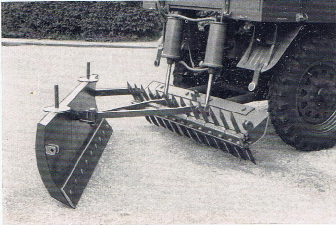
STRASSENPROFILIERGERÄT
