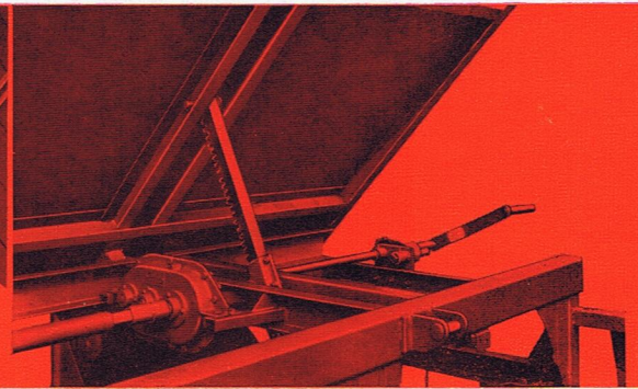
▲ Hintere Zahnstangenwinde mit staubdichtem Getriebe, Handkurbel mit Sicherheitsratsche und Rücklaufbremse
